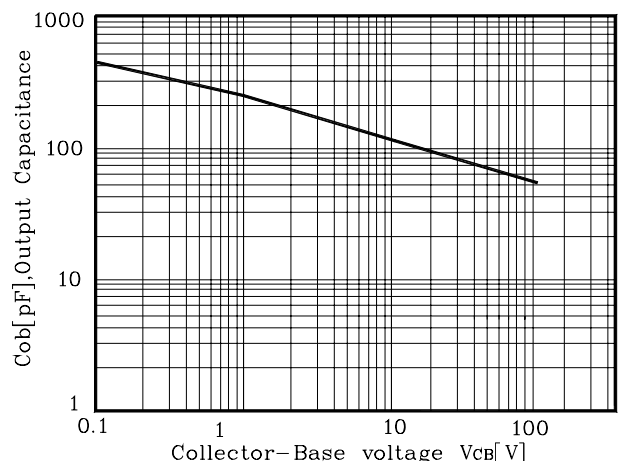
Fig. 6 C_{ob} - V_{CB}
